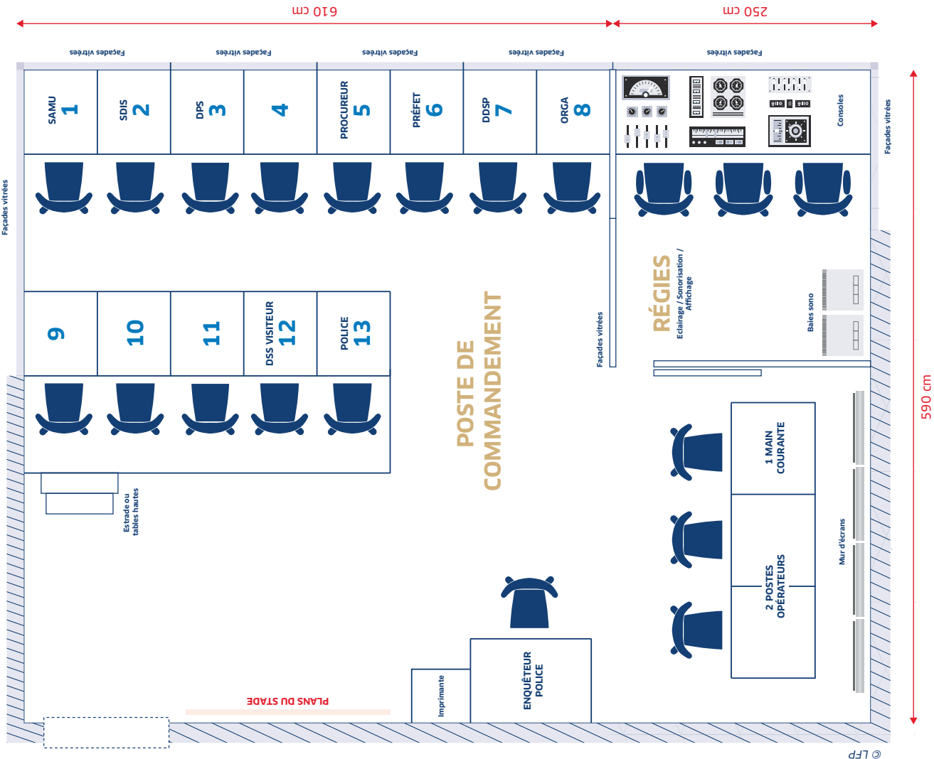
► Schéma n°36 : principe d'organisation du volume d'un PCM (dimensions conseillées)
